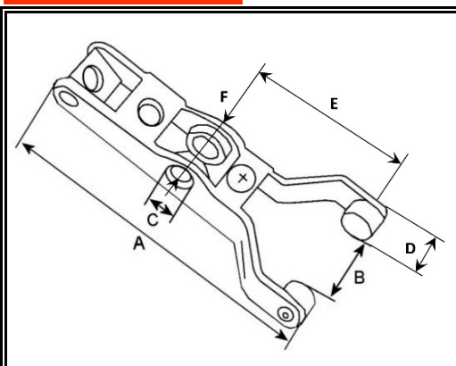
H1069 HORQUILLA DE ARRANQUE TIPO VALEO
